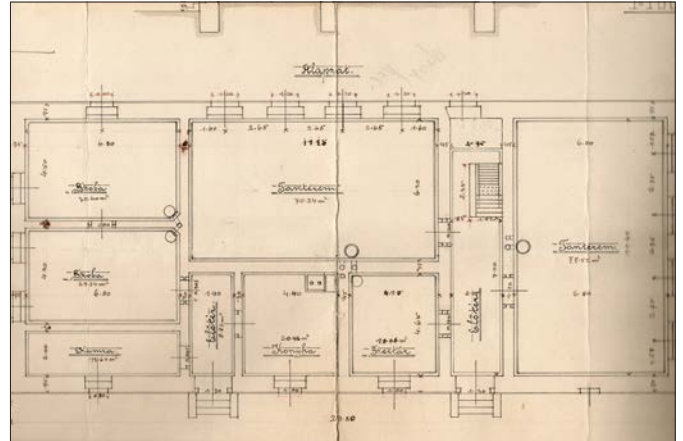
A Bajor kúria 1902-ben készült átalakítási terve, jelenleg ez az Ady Endre utca felőli épület
