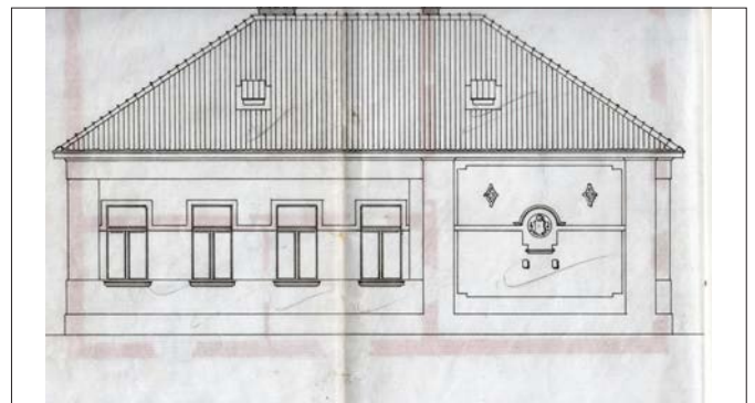
Szigetfő utcai felőli épület 1911-ben készült terve, utcai homlokzat
